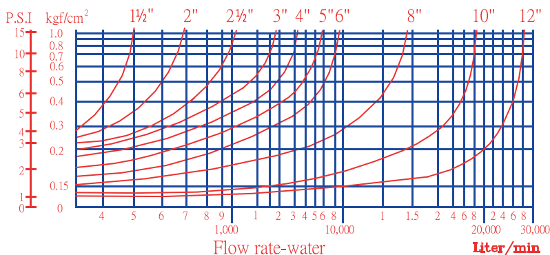
減壓閥流量參考曲線圖
