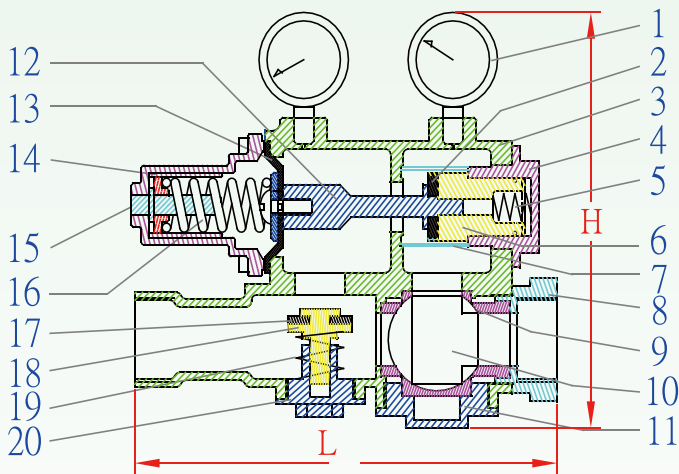
二次側壓力錶 一次側壓力錶
