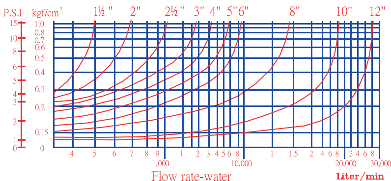
定水位閥流量參考曲線圖
