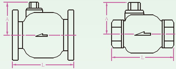
法蘭(BFF型)
