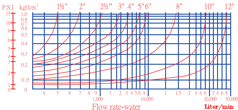
電磁閥流量參考曲線圖
