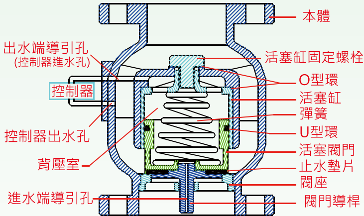
* 圖示為 常閉型 電磁閥
