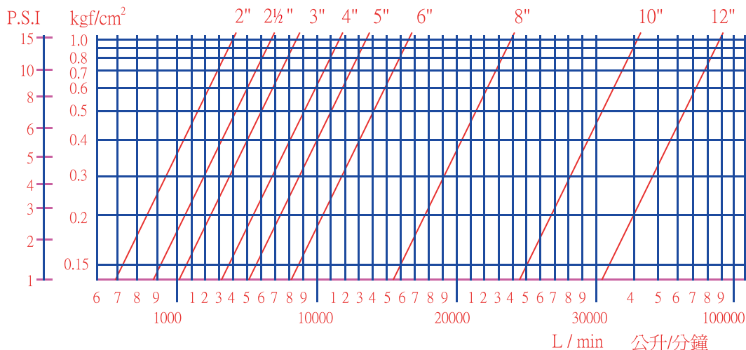
全開型靜音逆止閥流量曲線參考圖 Full Open Style Silent Check Valve Flow Chart
